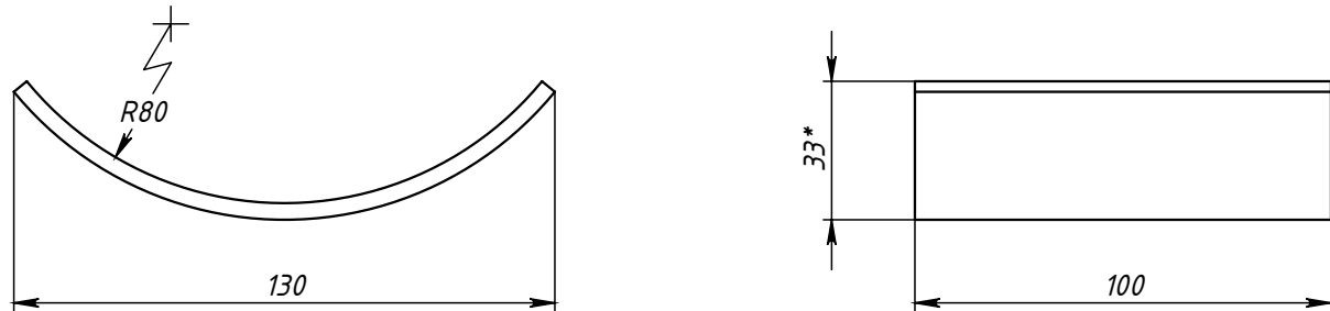
Поз.3 (Ложемент)
